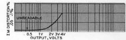
IM distortion.
